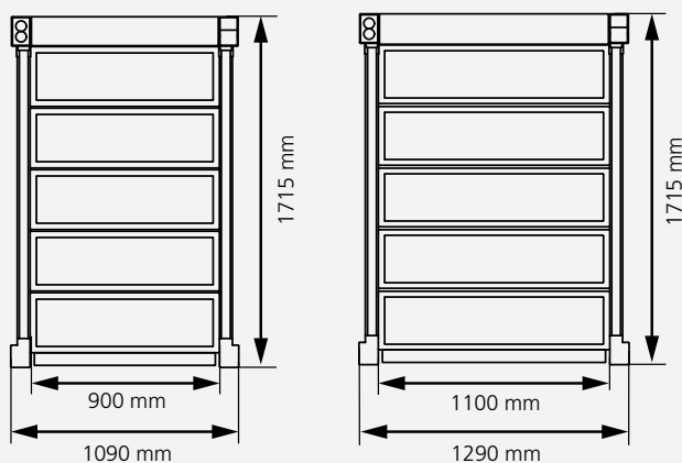
3-5 steg plattformslågen (mått)
