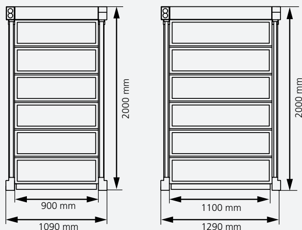
6 steg plattformslågen (mått)
